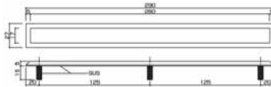
埋込工法 共通図面
