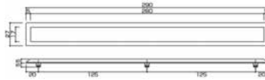
ホック式工法 共通図面
