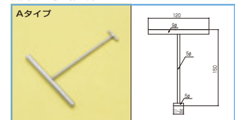
開閉取っ手 (在庫)
