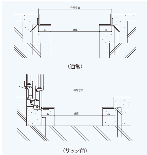
納まり図
