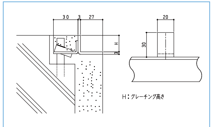
直角アンカー横付
