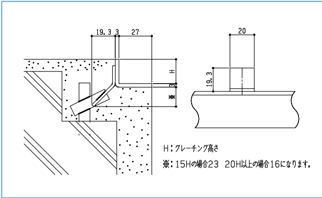
通常アンカー
