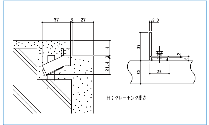
ホルダーアンカー
