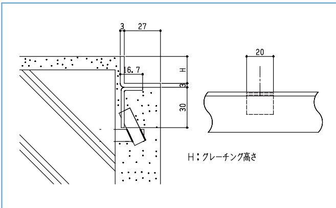
直角アンカー下付
